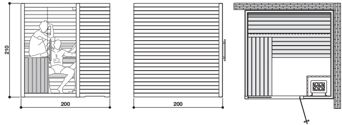
Vista versione Dx + 1 laterale Sx · View of RH version + 1 LH side Vue version D. + 1 panneau latéral G. · Ansicht: rechte Version + 1 linke Seite
