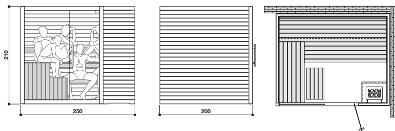
Vista versione Dx + 1 laterale Sx · View of RH version + 1 LH side Vue version D. + 1 panneau latéral G. · Ansicht: rechte Version + 1 linke Seite
