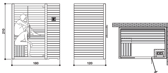
Vista versione Dx + 1 laterale Sx · View of RH version + 1 LH side Vue version D. + 1 panneau latéral G. · Ansicht: rechte Version + 1 linke Seite
