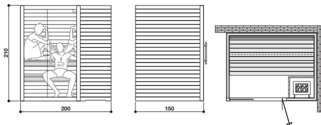
Vista versione Dx + 1 laterale Sx · View of RH version + 1 LH side Vue version D. + 1 panneau latéral G. · Ansicht: rechte Version + 1 linke Seite
