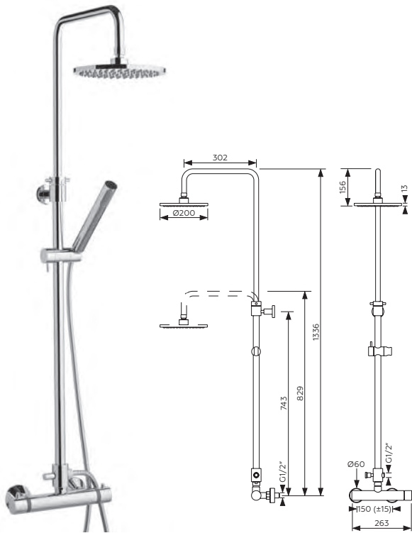
COLUNA DUCHE COM INVERSOR INTEGRADO SHOWER COLUMN WITH INTEGRATED DIVERTER COLONNE DOUCHE AVEC CONVERTISSEUR INTÉGRÉ
