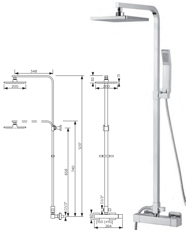
COLUNA DUCHE COM INVERSOR INTEGRADO SHOWER COLUMN WITH INTEGRATED DIVERTER COLONNE DOUCHE AVEC CONVERTISSEUR INTÉGRÉ
